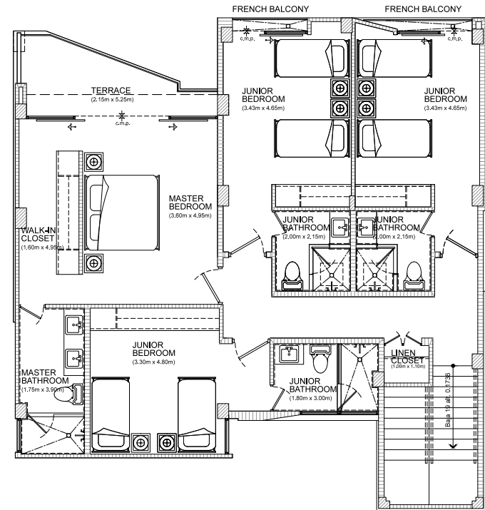
PLANTA ARQUITECTONICA NIVEL 100 SIN ESCALA
