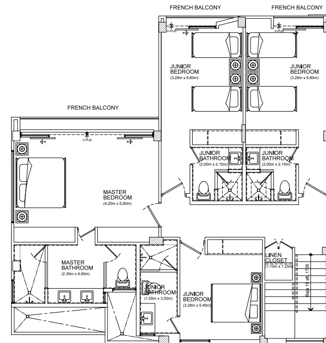
PLANTA ARQUITECTONICA NIVEL 100 - VILLA C SIN ESCALA
